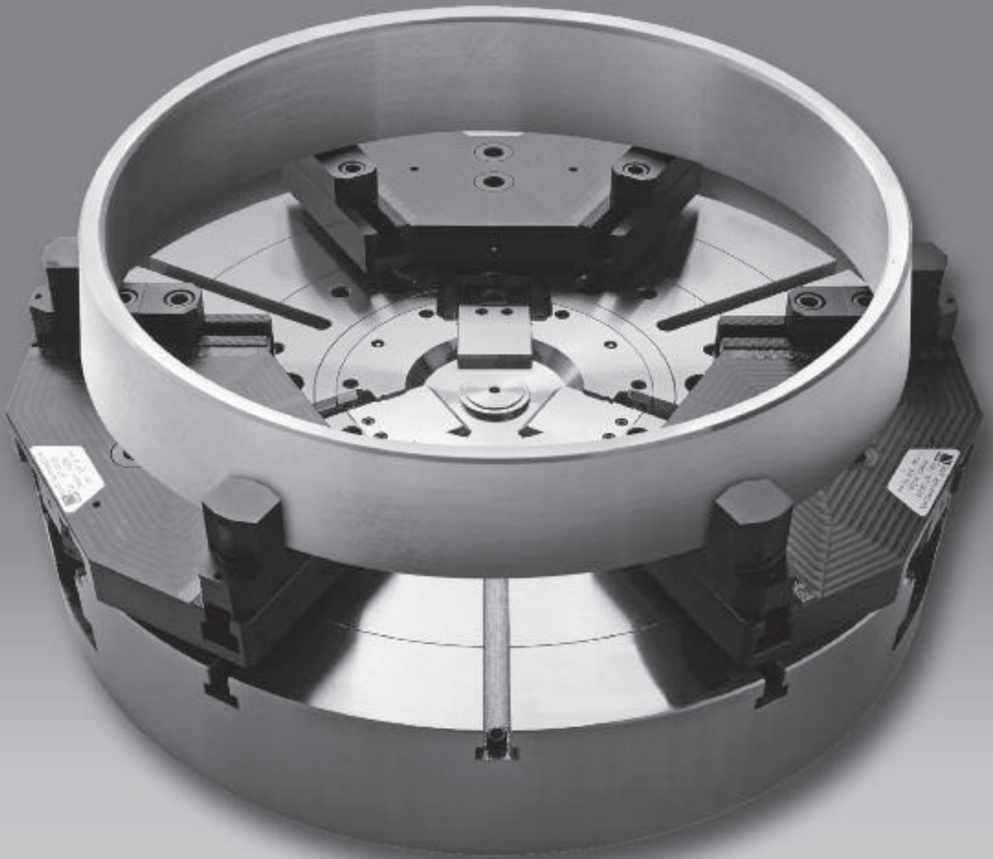
Inogrip Jaws
